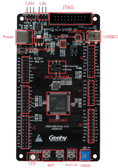
图 2 G32A1465 EVAL 底板
