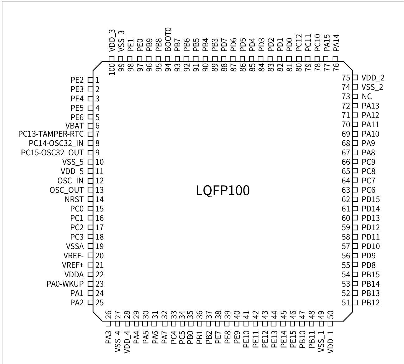
图2 LQFP100 引脚分布图
