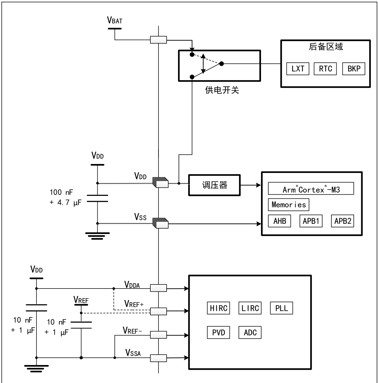
图10 供电方案
