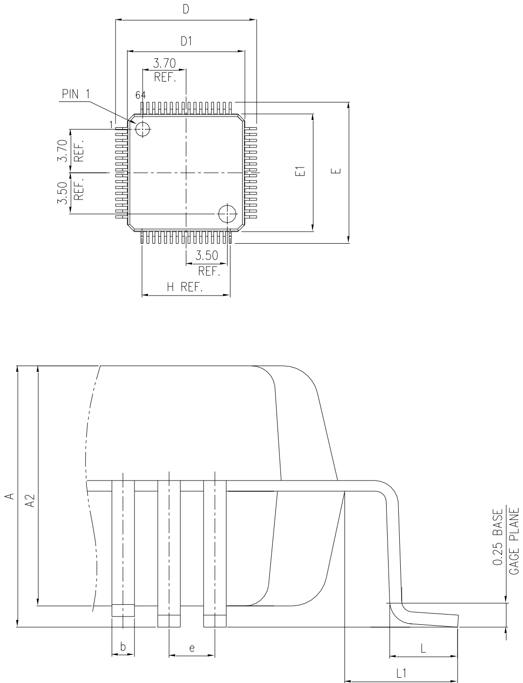
图24 LQFP64 封装图
