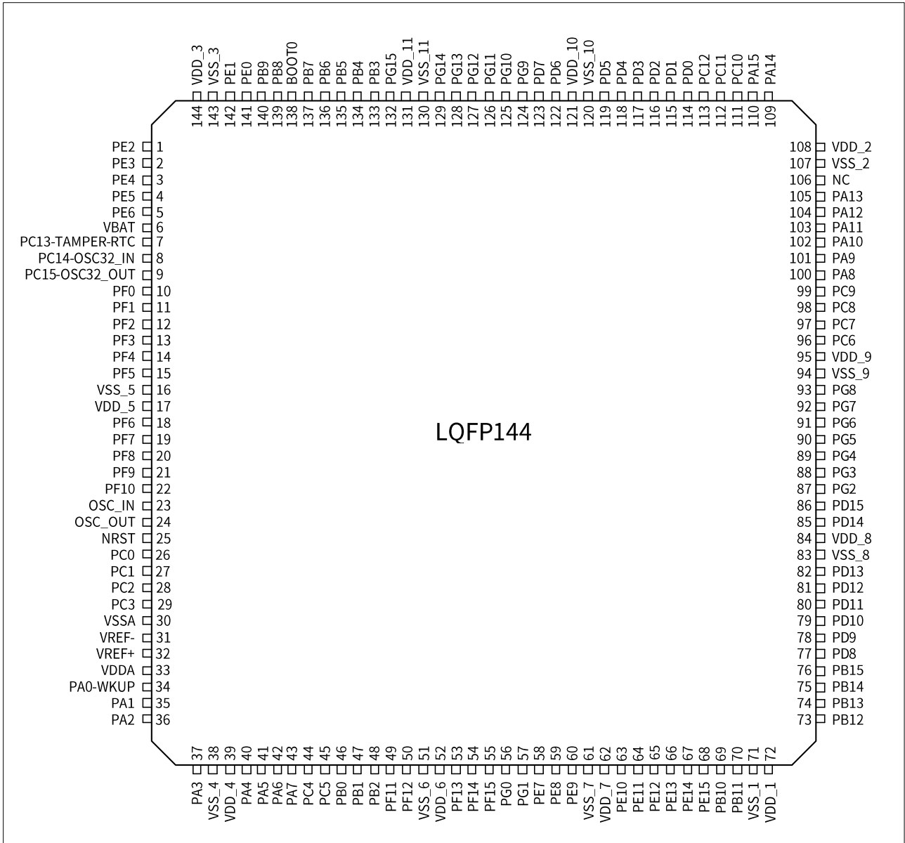
图1 LQFP144 引脚分布图
