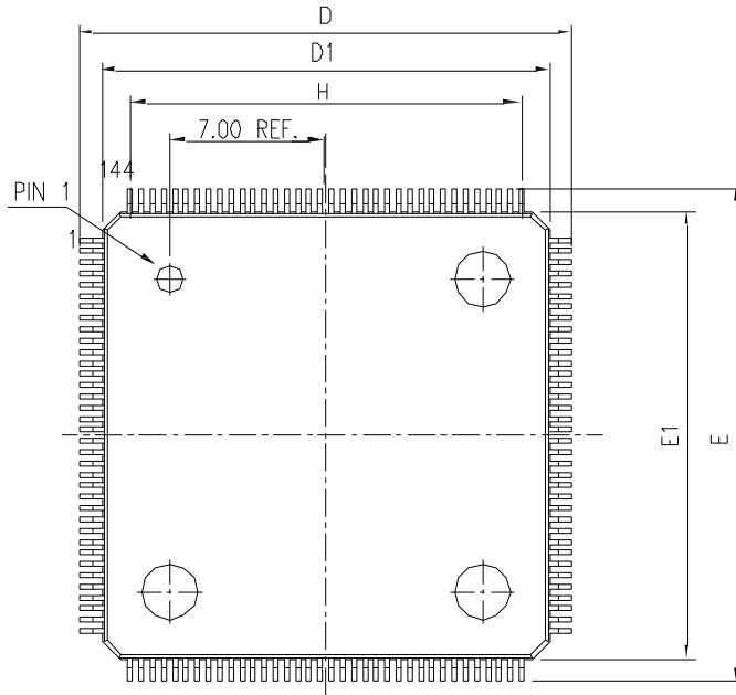
图18 LQFP144 封装图
