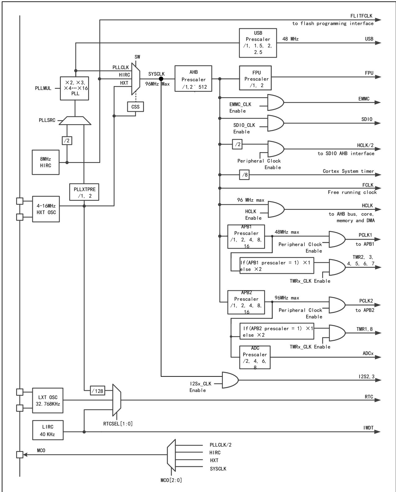
图5 APM32F103xCxDxE 系列时钟树
