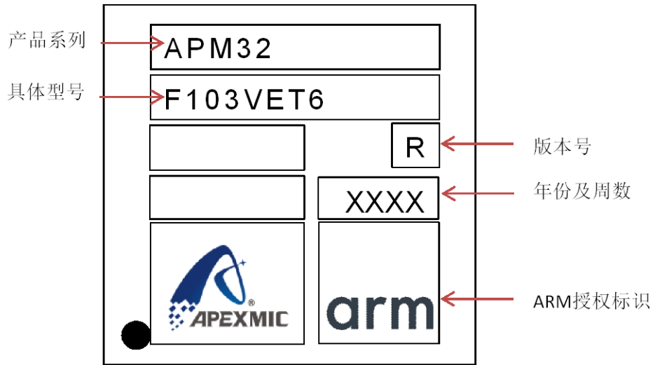
图23 LQFP100 - 100 引脚, 14 x 14mm 封装标识
