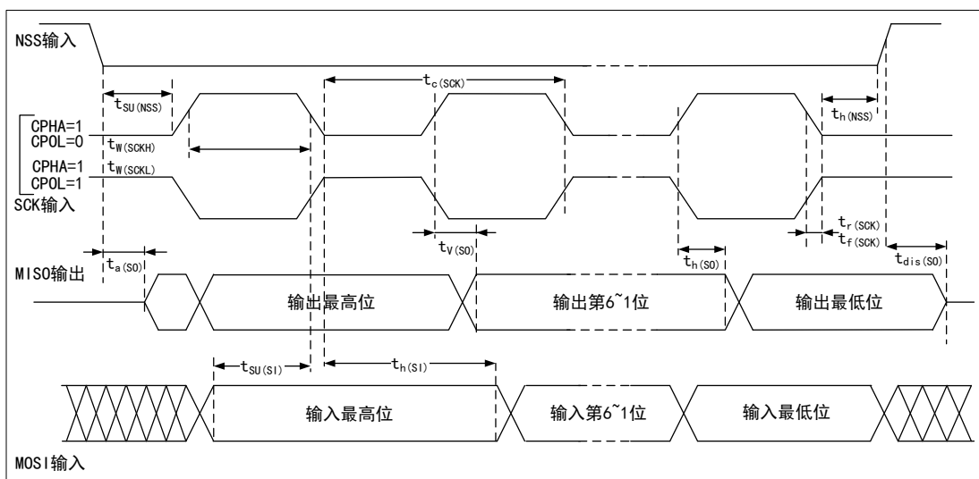
图17 SPI时序图 — 从模式和 CPHA=1(1)
