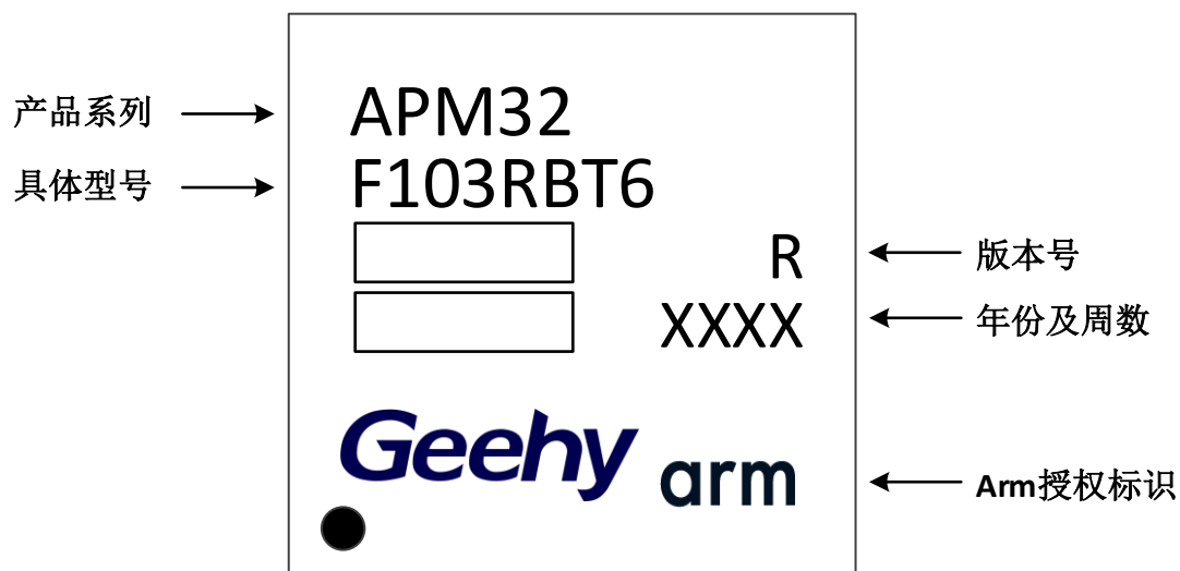
图27 LQFP64 - 64 引脚，10 x 10mm 封装标识
