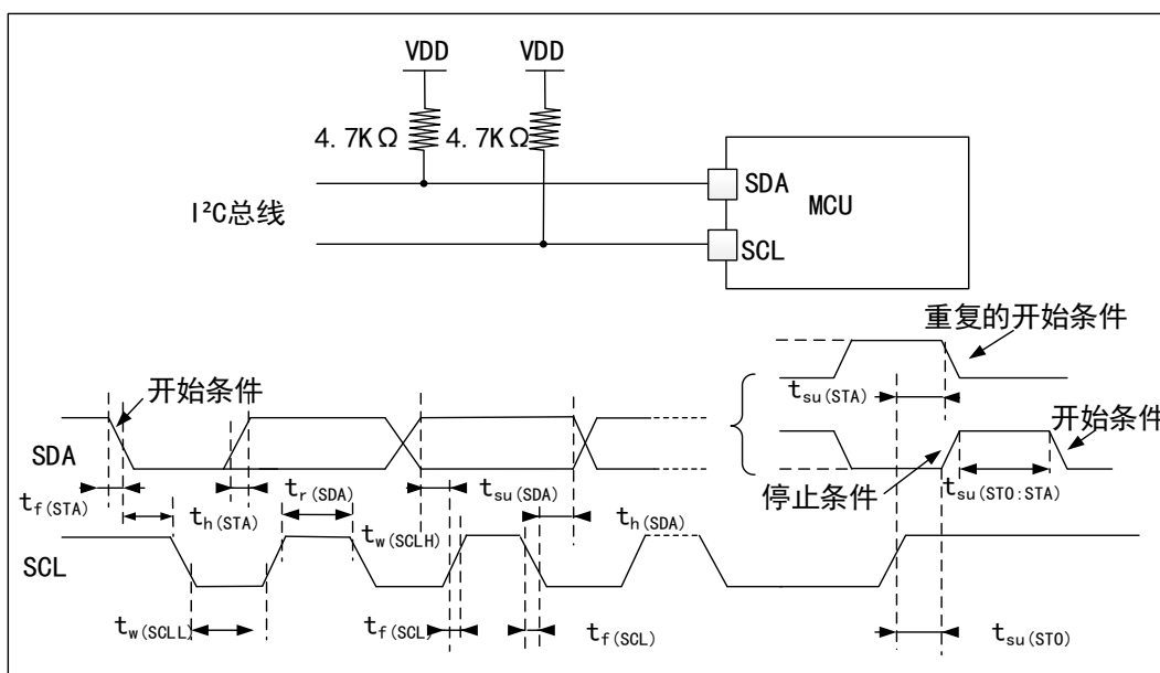
图15 总线交流波形和测量电路(1)
