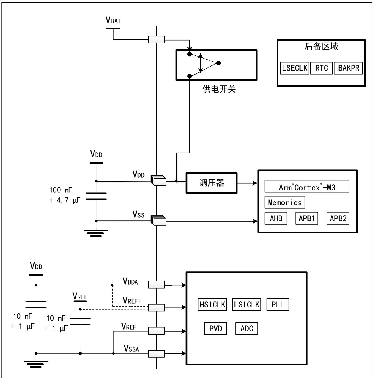
图8 供电方案
