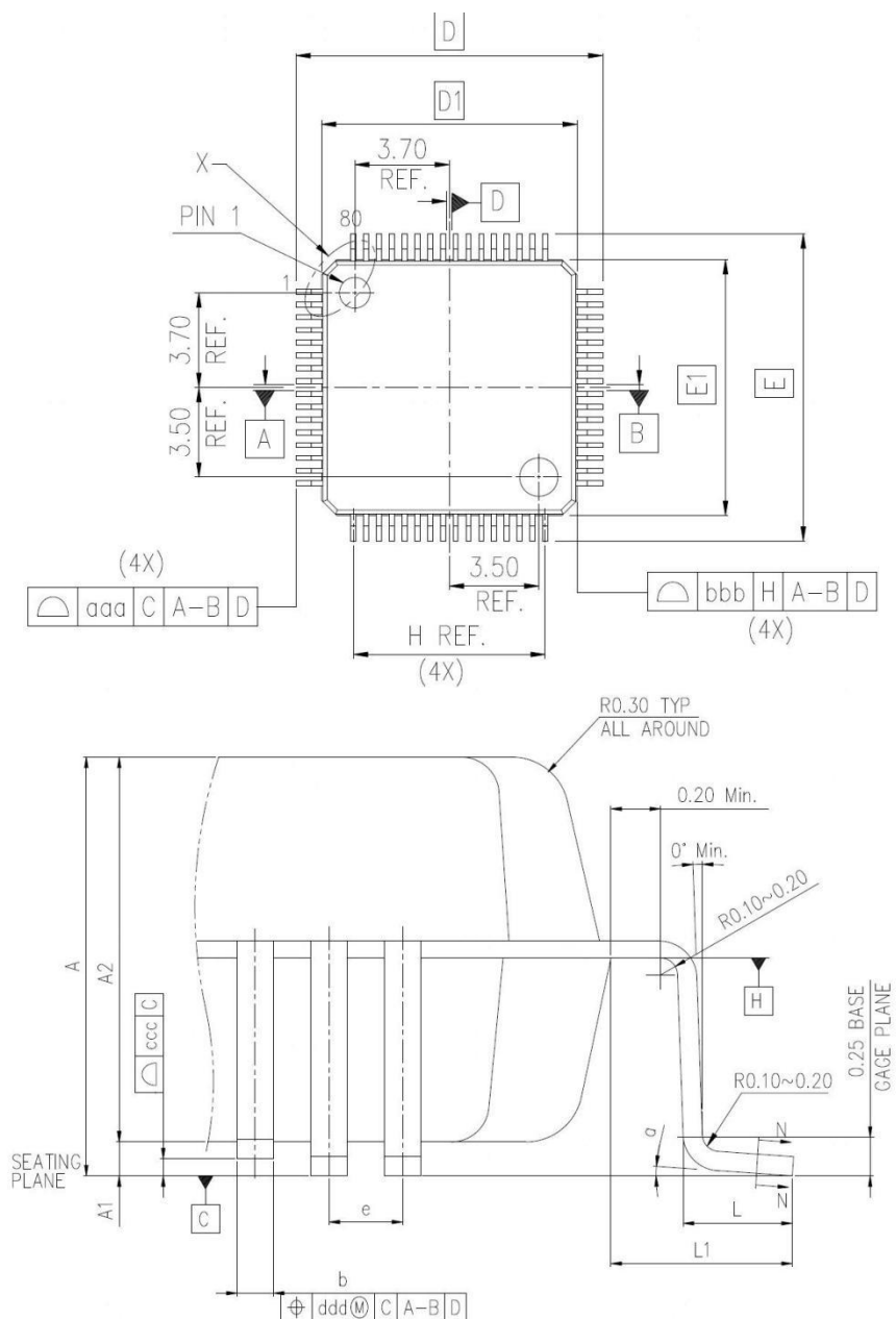
图25 LQFP64 封装图
