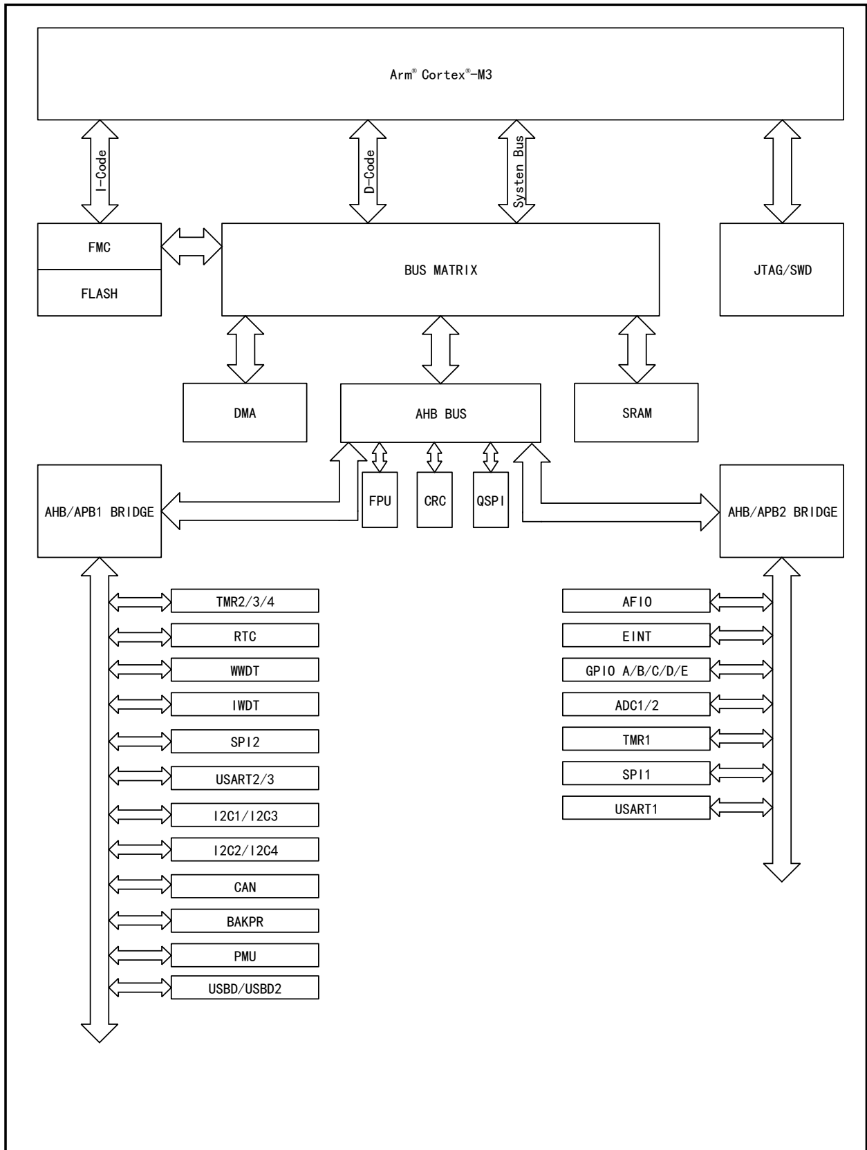
图5 APM32F103xB 系列系统框图
