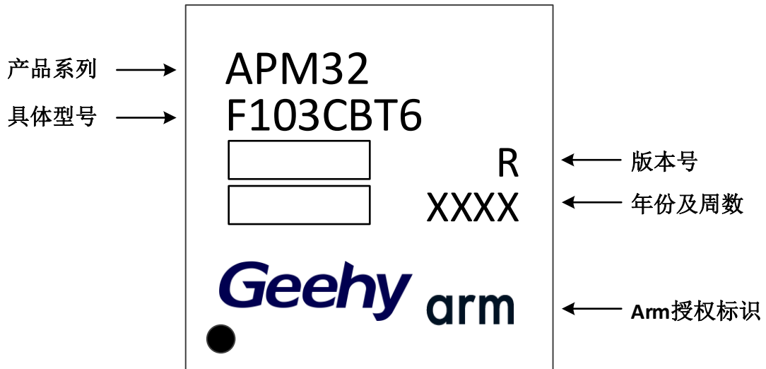
图30 LQFP48 - 48 引脚，7 x 7 mm 标识图
