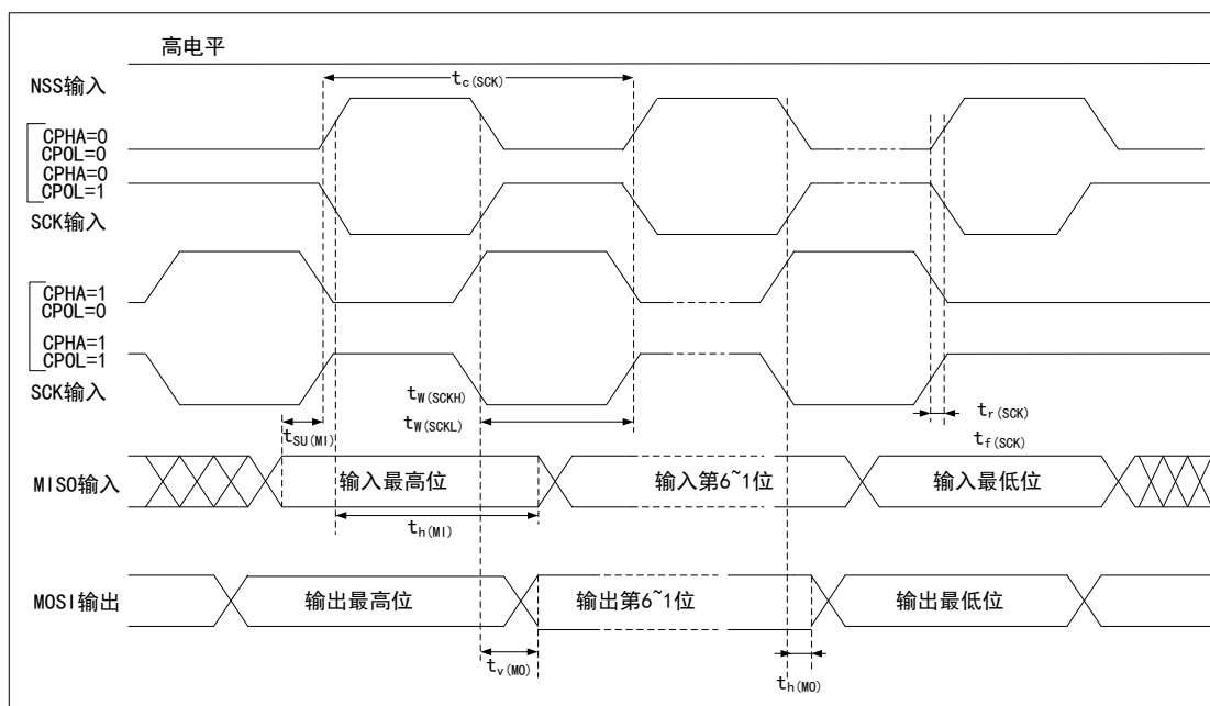
图18 SPI时序图 — 主模式(1)
