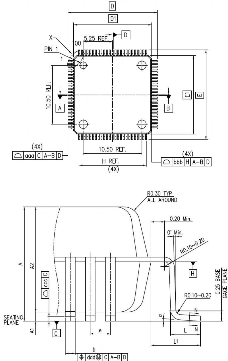
图22 LQFP100 封装图
