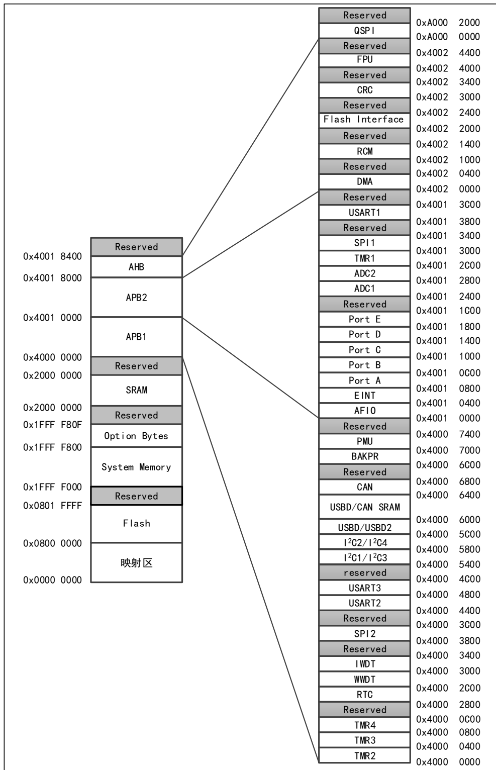
图7 APM32F103xB 系列地址映射图
