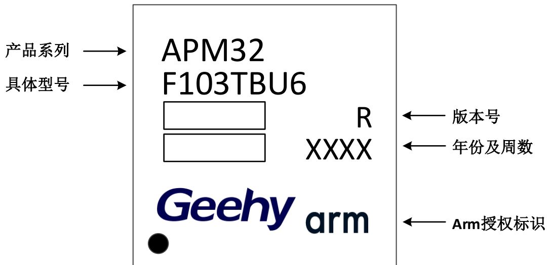
图33 QFN36 - 36 引脚，6 x 6 mm 标识图
