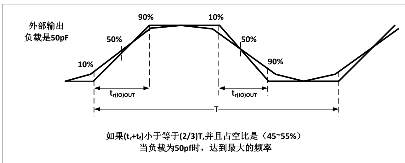
图14 输入输出交流特性定义
