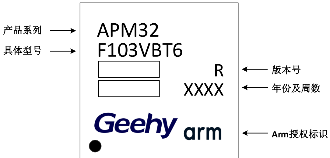
图24 LQFP100 - 100 引脚，14 x 14mm 封装标识
