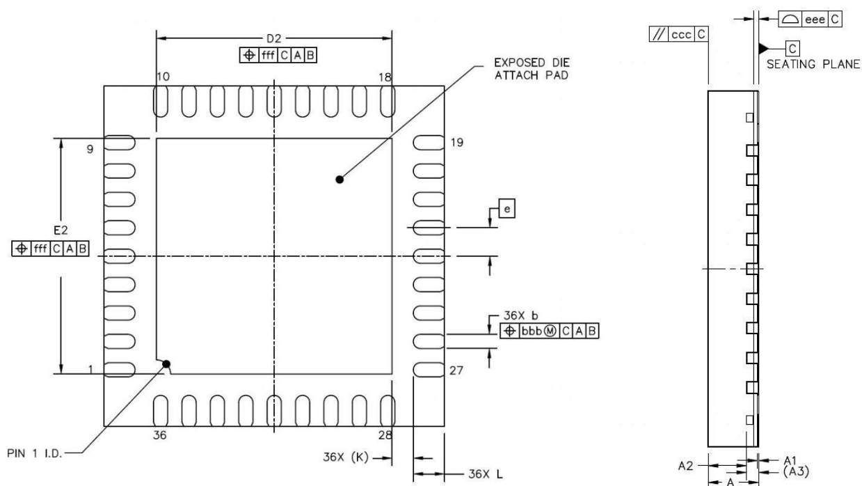
图 21 QFN36 封装图
