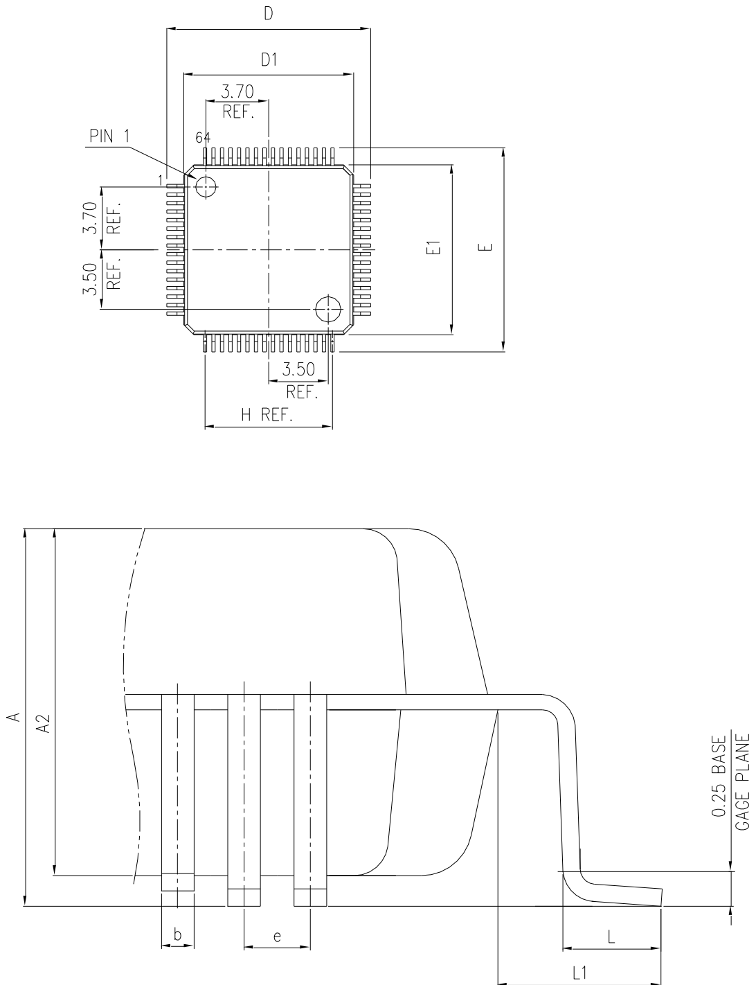
图 15 LQFP64 封装图
