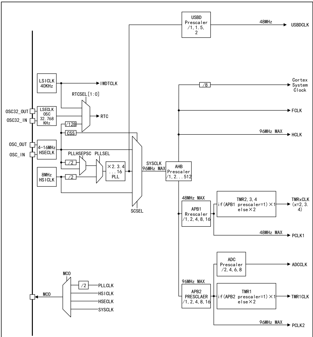
图 5 APM32F103x4x6x8 时钟树
