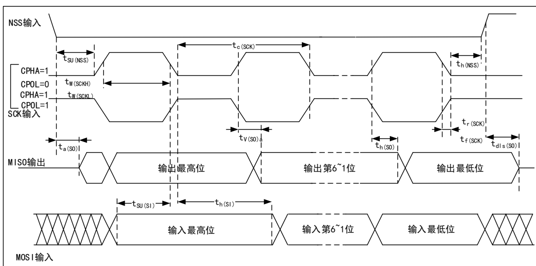
图10 SPI 时序图—从模式和 CPHA=1 (1)
