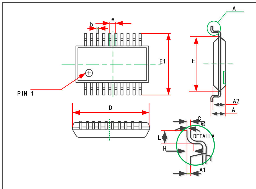
图12 TSSOP20 封装图
