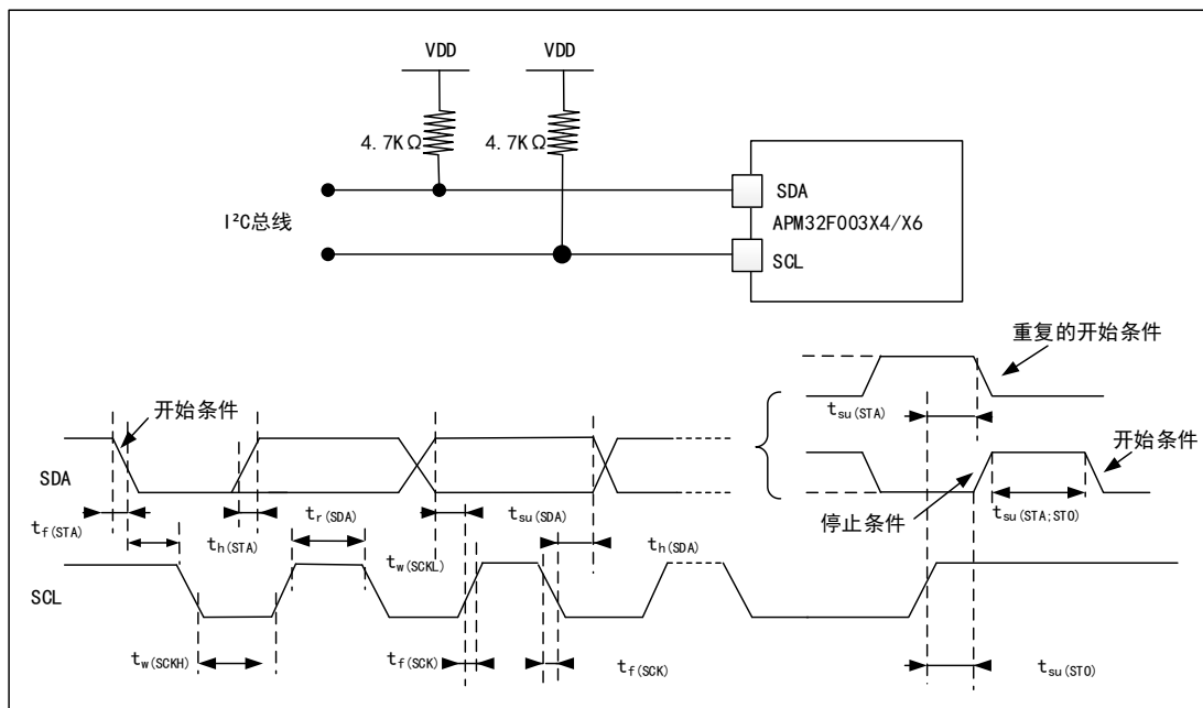
图8 总线交流波形和测试电路
