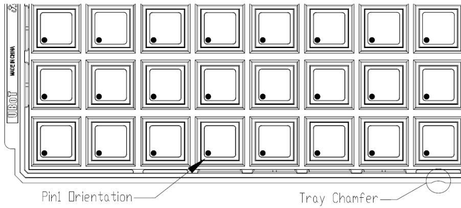
图18 Pin1 方向和托盘倒角
