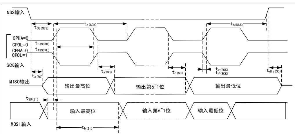
图9 SPI 时序图—从模式和 CPHA=0
